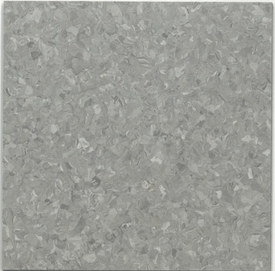
2603 Cineos
