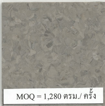
2615 Linear
