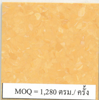
2609 Lemmon
