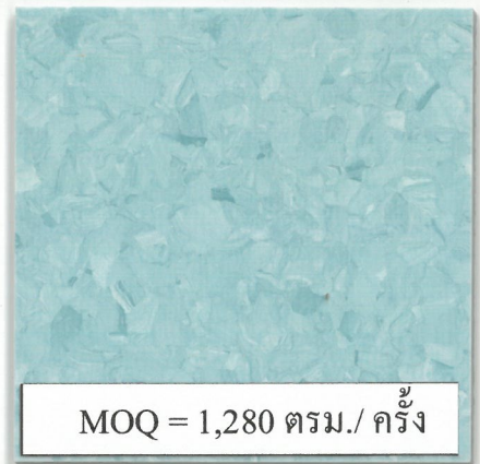
2611 Tritton
