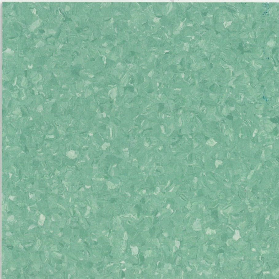
2625 Iras
